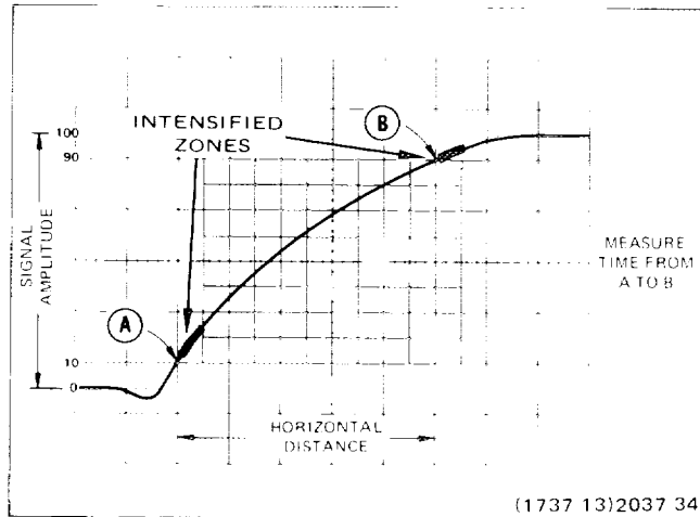
Fig. 34. Risetime.
