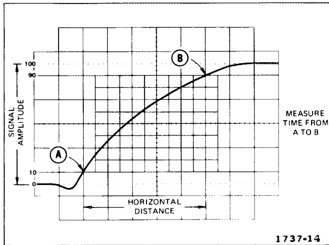
Fig. 21. Risetime.
