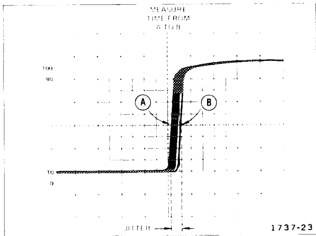
Fig. 25. Pulse jitter.
