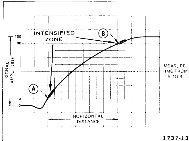
Fig. 30. Risetime.
